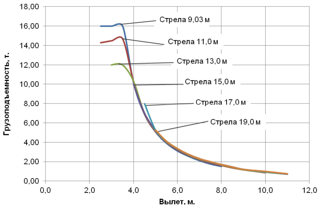
Рисунок 8 – Грузоподъемность без противовеса. Зона работы 360°
